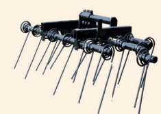
3-soros, 3-részes pálcás elmunkáló, Ø16 mm-es pálcákkal
